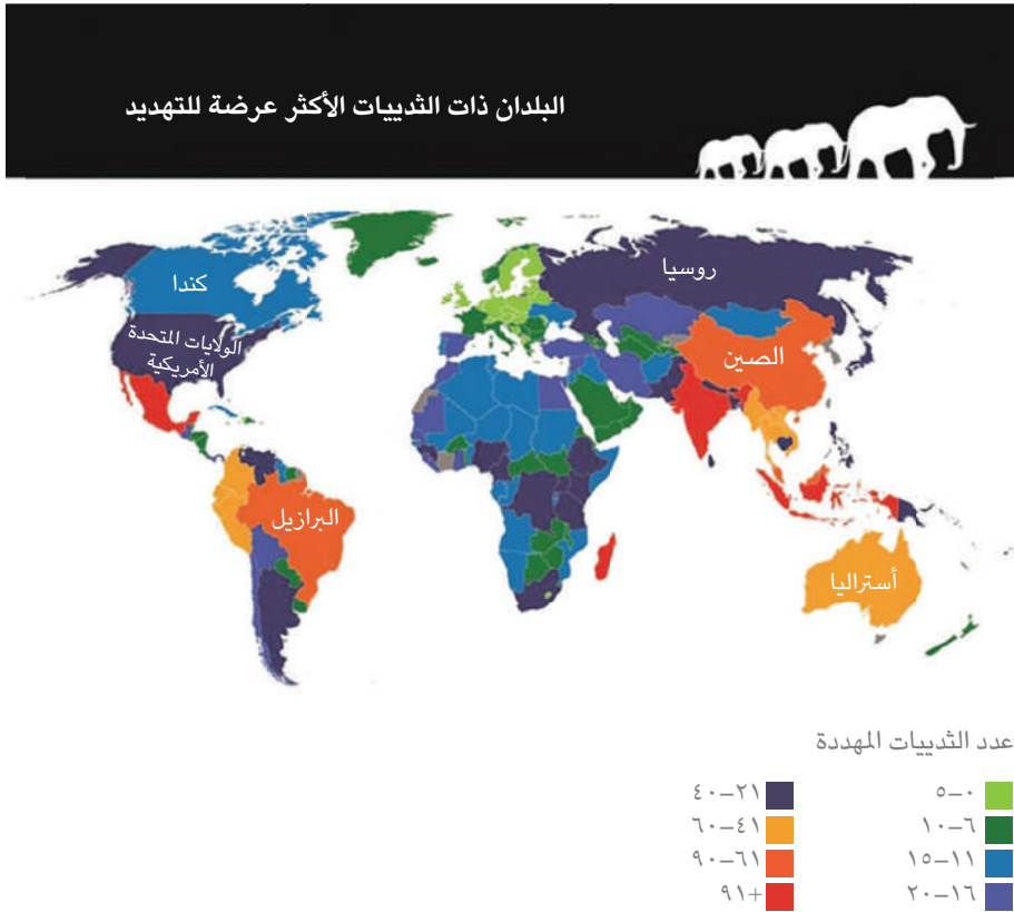
شكل ٢-١: البلدان ذات الثدييات الأكثر عرضة للتهديد. (المصدر: www.theecoexperts.co.uk ، بيانات من البنك الدولي.)
