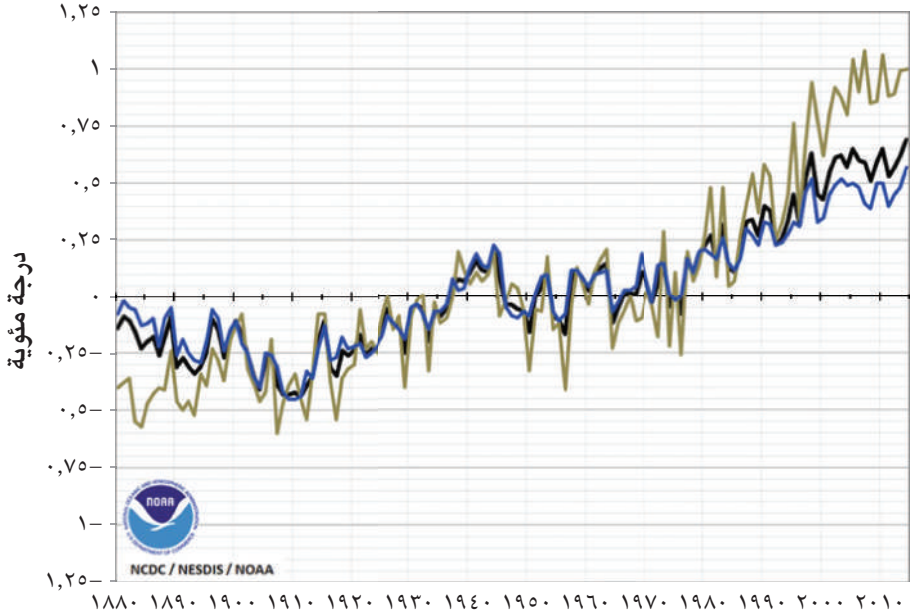
درجة الحرارة السنوية العالمية (للأرض والمحيط والاثنين مجتمعين)
