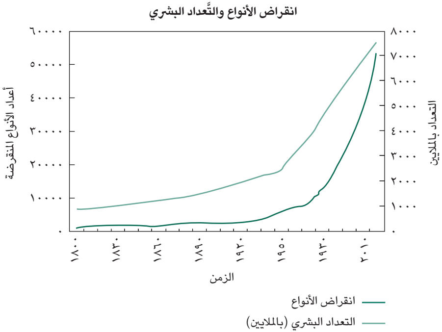
شكل ٢-٣: انقراض الأنواع والتَّعداد البشري. (المصدر: هيئة المسح الجيولوجي الأمريكية، ٢٠٠٨).
