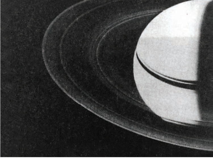
شكل ٧-٢٠: زحل. سفينة الفضاء فوياجر ٢ مرّت عبر كوكب زحل في أغسطس ١٩٨١ م. وكشفت الصور عن تفاصيل مذهلة غير معروفة عن الهالة الجميلة المحيطة بالكوكب.
