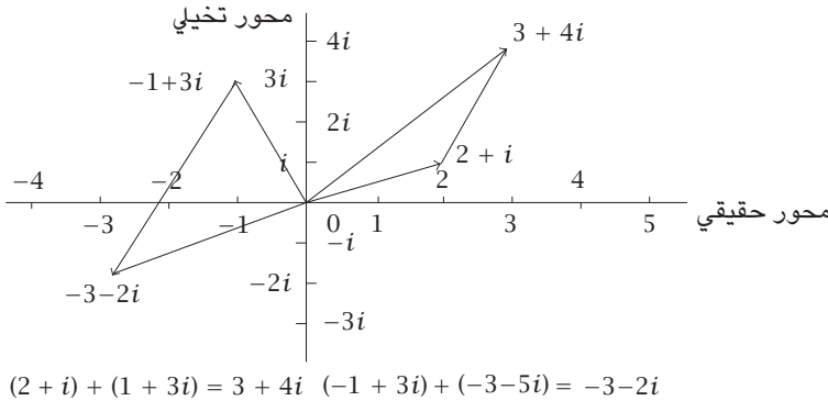
شكل ٨-١: إضافة الأعداد المركبة عن طريق إضافة قطع مستقيمة موجهة.
