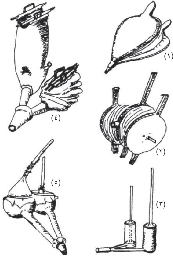
شكل ٦-٢: أنواع الكور البدائية (منفخ الهواء): (١) و (٢) منفخ أكورديون. (٣) منفخ بستون. (٤) و (٥) منفخ جلدي فخاري.
