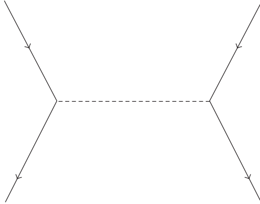
شكل ٩-٩: في شكل فاينمان يتفاعل جسيمن بأن يتبادلا جسيماً ثالثاً. وفي هذه الحالة تحديداً من الممكن أن يكون الجسيمن إلكترونين يتبادلان فوتوناً ويتنافران أحدهما مع الآخر.
