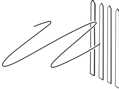
شكل ١٠-٢: حجب موجات مستقطبة أفقيًا.
