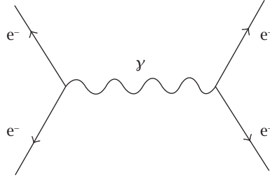
شكل ١: مخطط فاينمان الكلاسيكي لتفاعلات الجسيم.
