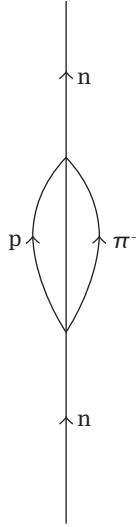
شكل ٩-١٩: يمكن أن يتحوّل نيوترون لفترة وجيزة إلى بروتون زائد بيون مشحون على أن يعود الاثنان معاً بسرعة.
