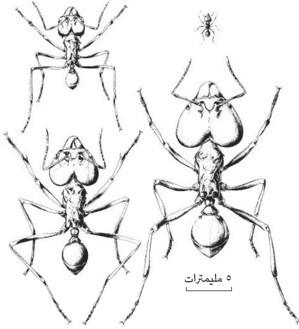
شكل ٧-٢: طبقات النمل الشغالة في مجموعة النمل القاطعة للأوراق المعروفة باسم «أنا»، وكلها من المستعمرة عينها. الشغالة الصغيرة بأعلى اليمين تعتني بحدائق الفطريات التي يزرعها هذا النوع، أما النملات العملاقة فهي الجنود، التي تحرس العش.
