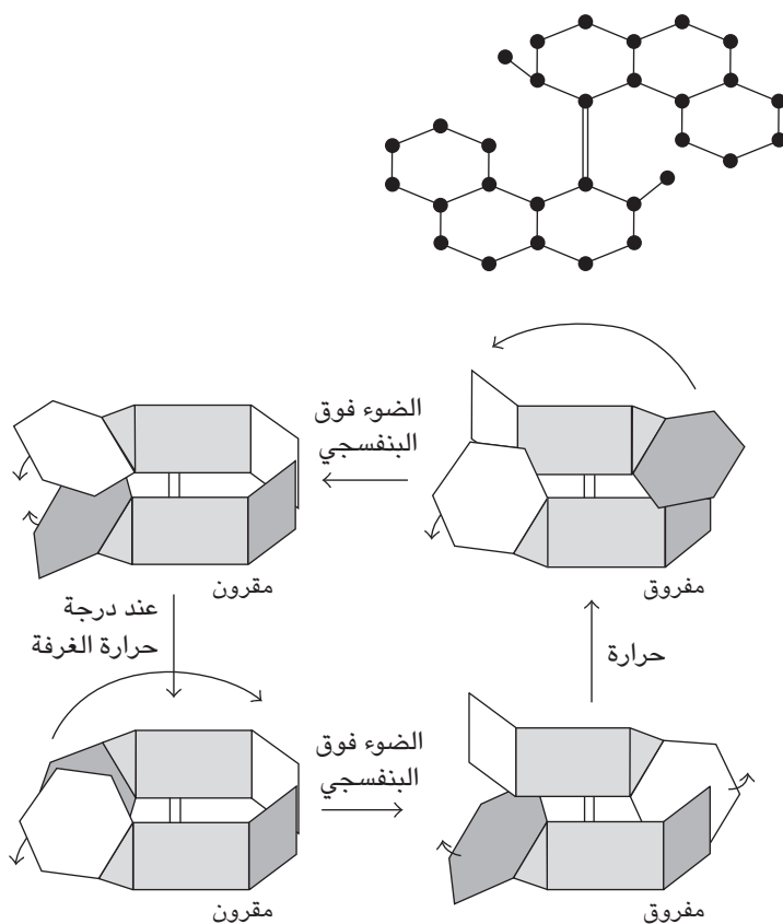
شكل ٥-٦: محرك جزيئي دوار مصنوع من الصفر، ويشتغل بالطاقة الضوئية. تُظهر الصورة العليا هيكل ذرات الكربون.
