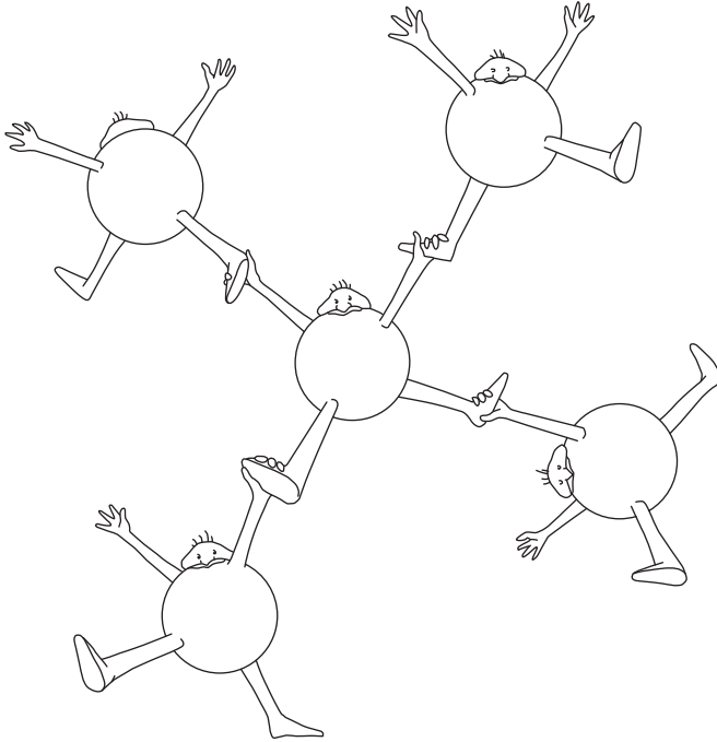
شكل ١-٣: إنَّ جَعَلَ الجزيئات تبدو في صورة بشرية يمكن أن يفيد في رؤية كيفية تفاعلها فيما بينها. وفي هذا الشكل أظهر «مسكات الأيدي» الضعيفة التي توجد فيما بين جزيئات الماء.
