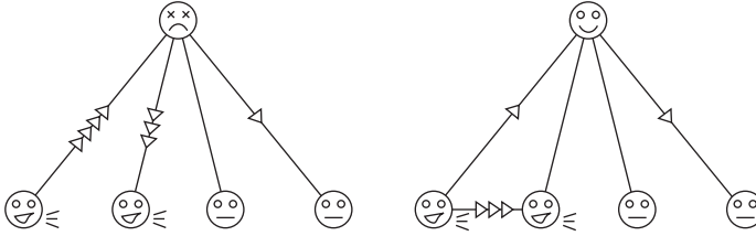
شكل ٩-٣: خوارزمية مثالية محليًا. يتم تجاوز نقطة التلاقي الأكثر ازدحامًا عن طريق إضافة رابط بين النقطتين المجاورتين اللتين يُرسل إليهما معظم الرسائل (المشار إليهما بالأسم).
