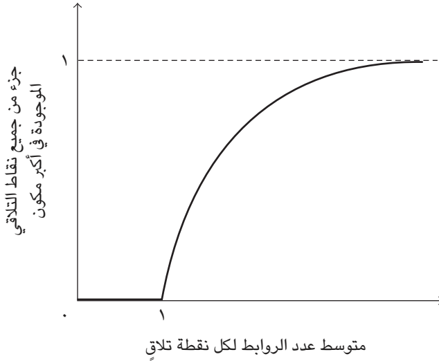
شكل ٢-٢: اتصالية الرسم البياني العشوائي. يتغير عدد نقاط التلاقي المتصلة في مكون واحد فجأة عندما يتجاوز متوسط عدد الروابط لكل نقطة تلاقٍ واحدًا.
