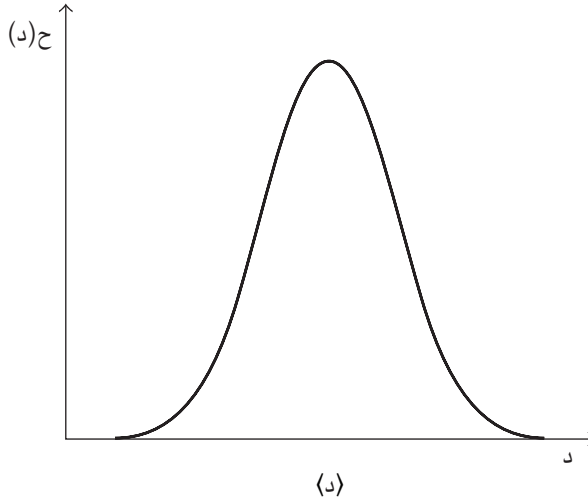
شكل ٤-١: يحدد التوزيع الطبيعي احتمالية ح(د) أن يكون لدى نقطة تلاقٍ واحدة مُختارة عشوائياً عدد (د) من الجيران. وتقع الدرجة المتوسطة (د) بقمة التوزيع.
