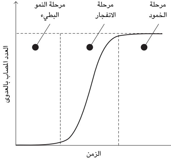
شكل ٦-٤: النمو اللوجستي، الذي يوضح مرحلة النمو البطيء ومرحلة الانفجار ومرحلة الخمود.
