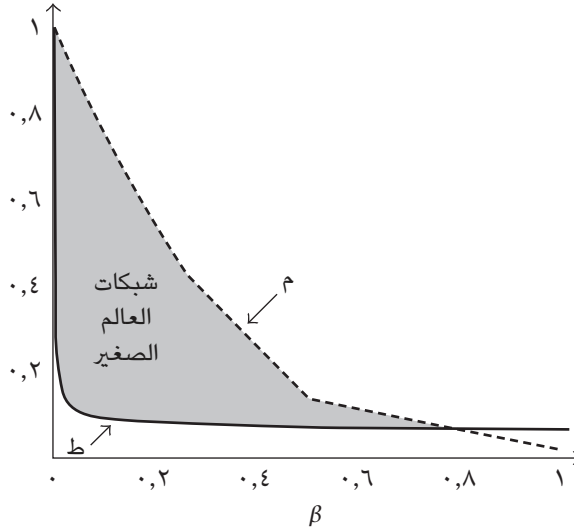
شكل ٣-٧: طول المسار ومعامل التكتل في النموذج بيتا. كما هو الحال مع النموذج ألفا (انظر الشكل ٣-٤)، تظهر شبكات العالم الصغير عندما يكون طول المسار صغيراً ومعامل التكتل كبيراً (المنطقة المظللة).
