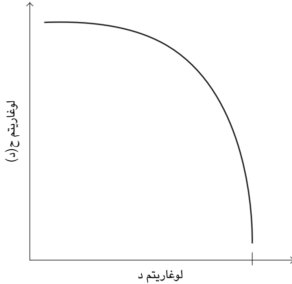
شكل ٤-٤: توزيع طبيعي على بياني لوغاريتم-لوغاريتم. يحدث «القطع» عندما يختفي المنحنى داخل المحور الأفقي.
