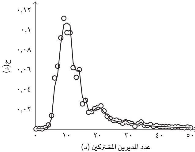
شكل ٧-٤: توزيع المديرين المشتركين وفق بيانات مجالس الإدارات التي تناولها الشبكة، كما هو موضح فيجبري ديفيز. الدوائر هي البيانات الحقيقية، والخط هو التوقع النظري.
