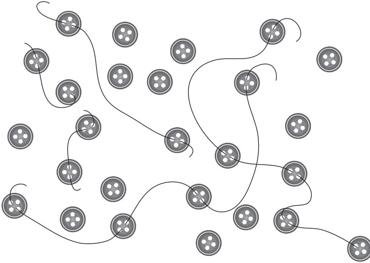
شكل ٢-١: رسم بياني عشوائي مُتخيل يصور مجموعة من الأزوار المربوطة معًا بخيوط. تتصل أزواج من نقاط التلاقي (الأزوار) معًا عشوائيًا عن طريق روابط أو صلات.
