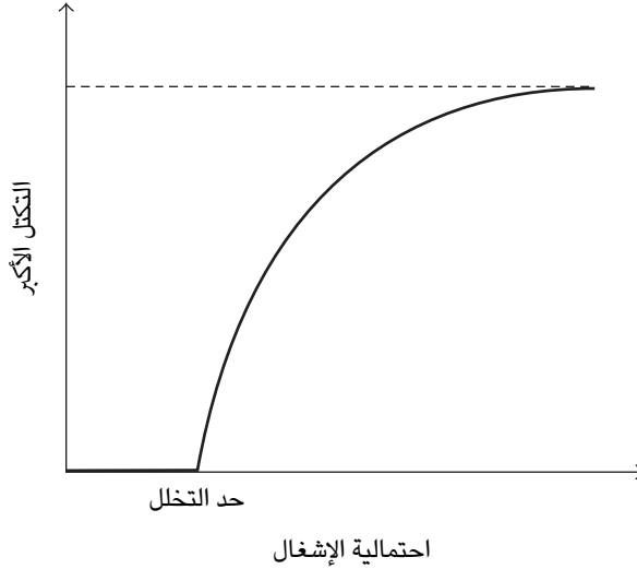
شكل ٦-١٢: أكبر تكتل قابل للعدوى في إحدى الشبكات. يشغل التكتل الأكبر، فوق حد التخلل، جزءاً محدوداً من الشبكة، مما يشير إلى أن ظهور المرض يمكن أن يصير وباءً.
