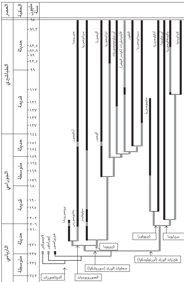
شكل ٤-١: مخطط الفرع الحيوي للديناصورات.
