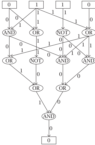
شكل ١-٤: برنامج كمبيوتر بسيط
