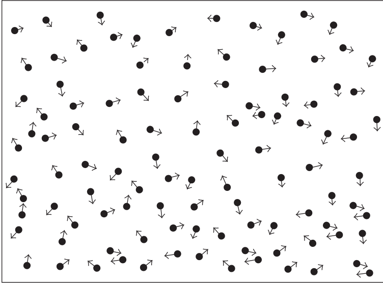
شكل ١-٣: نموذج ثنائي الأبعاد لأحد الغازات
