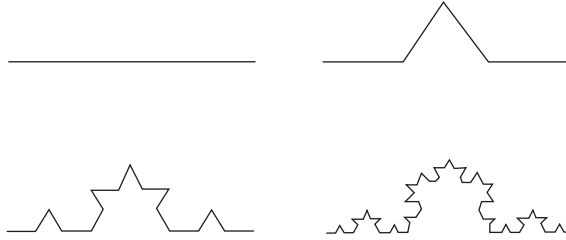
شكل ٥-٥: إنشاء منحنى ندفة الثلج لكوخ
