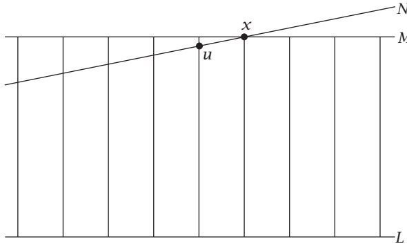
شكل ٦-٤: أحادية المستقيمت المتوازية
