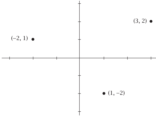
شكل ٥-١: ثلاثة نقاط في المستوى الديكارتي
