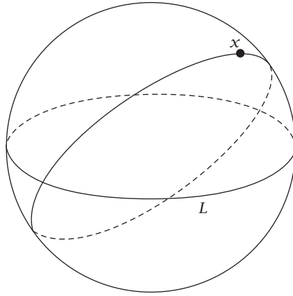
شكل ٦-٦: لا تنطبق مُسَلِّمة التوازي على الهندسة الكروية
