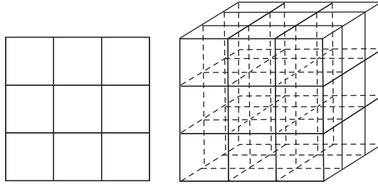
شكل ٥-٤: تقسيم مربع إلى عدد 9 = 3^2 من المربعات الأصغر، وتقسيم مكعبٍ إلى عدد 27 = 3^3 من المكعبات الأصغر
