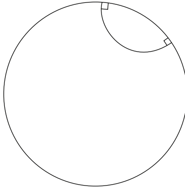
شكل ٦-٩: مستقيمٌ زائدي نموذجي
