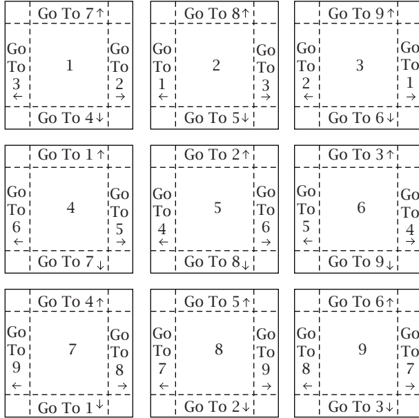
شكل ٦-١٣: أطلس لطارة (سطح حلقي)
