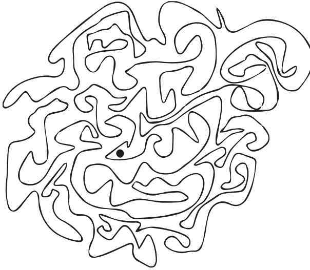
شكل ٣-٩: هل تقع النقطة السوداء داخل المنحنى أم خارجه؟
