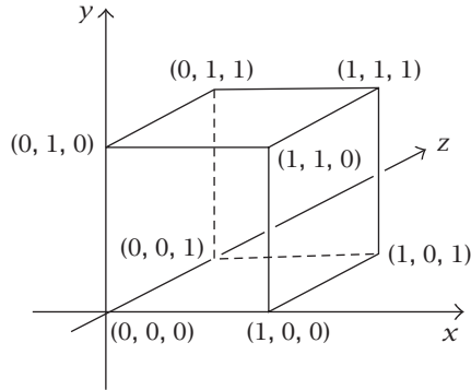
شكل ٥-٣: مربع الوحدة ومكعب الوحدة
