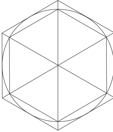
شكل ٣-٤: إيجاد مساحة دائرة تقريبياً بواسطة مضلع
