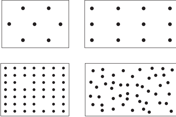
شكل ٢-٣: طرق تمثيل الأعداد 7 و 12 و 47 (مرتين)
