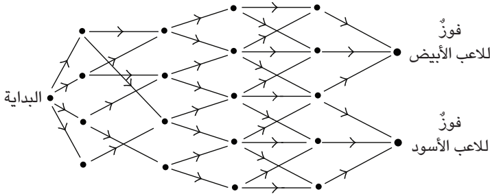
شكل ١-٢: بداية المباراة عند اللاعب الأبيض، ولديه استراتيجية رابحة
