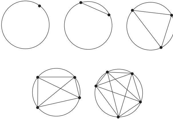
شكل ٣-١: تقسيم دائرة إلى أجزاء
