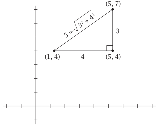
شكل ٥-٢: حساب المسافات باستخدام نظرية فيثاغورس
