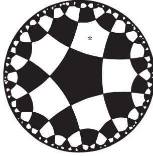
شكل ٦-٨: تغطية مستوًى زائديّ بأشكالٍ خماسية منتظمة
