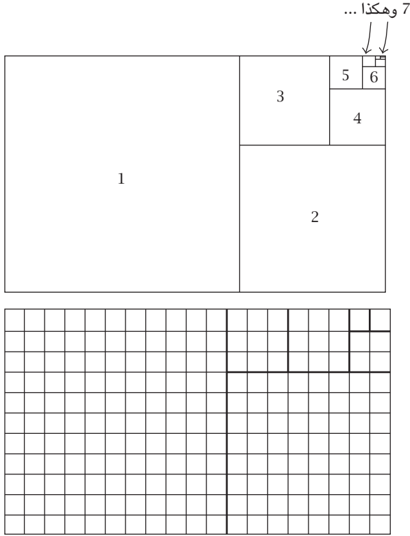
شكل ٣-٣: اقتطاع مربعاتٍ من مُستطيلات
