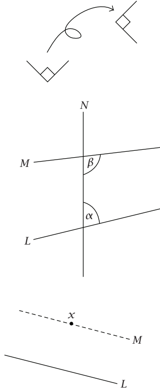
شكل ٦-١: المسلّمة الرابعة لإقليدس ومثالان على المسلّمة الخامسة
