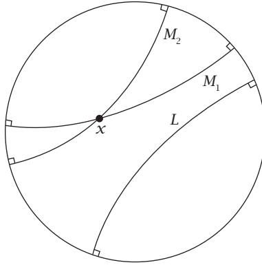
شكل ١١-٦: مسلَّمة التوازي لا تتحقق في المستوى الزائدي
