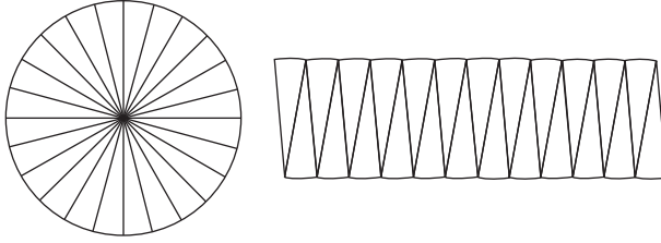
شكل ٤-٢: طريقة أرشميدس لإثبات أن مساحة الدائرة تساوي \pi r^2
