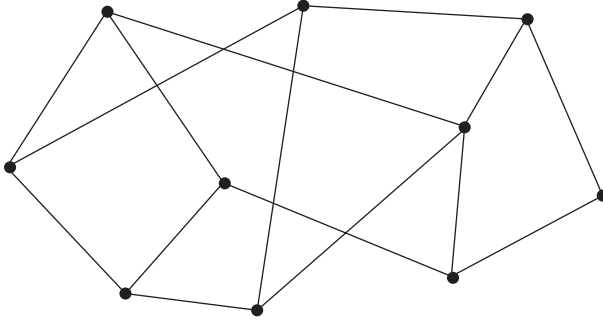
شكل ١-٥: رسم له ١٠ رؤوس، و ١٥ ضلعًا
