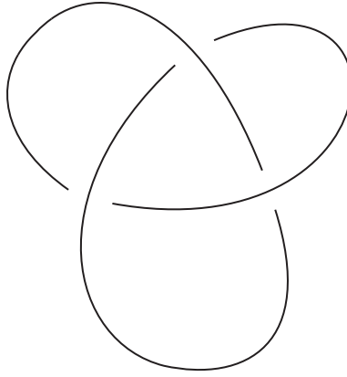
شكل ٣-٧: عقدة ثلاثية الؤريقات
