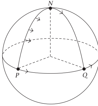
شكل ٦-٧: العبارة «في الاتجاه نفسه» لا معنى لها على سطح الكرة
