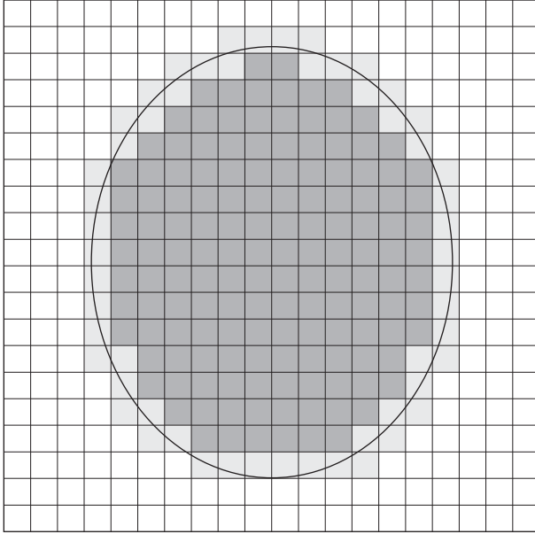
شكل ٤-١: حساب المساحة التقريبية لشكل منحنٍ
