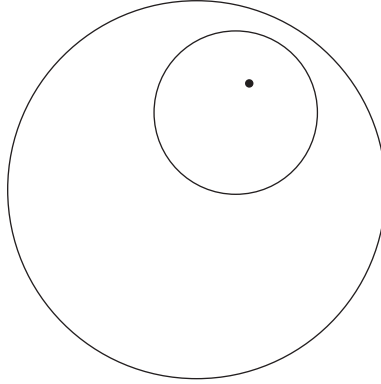
شكل ٦-١٠: دائرة زائدية نموذجية، ومركزها
