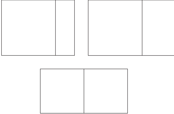
شكل ٣-٢: وجود النسبة الذهبية
