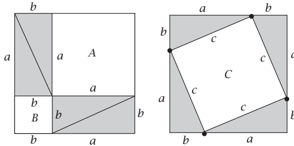
شكل ٣-٥: برهان مُوجز لنظرية فيثاغورس
