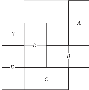
شكل ٣-٦: تغطية شبكة من المربعات بإزالة الأركان
