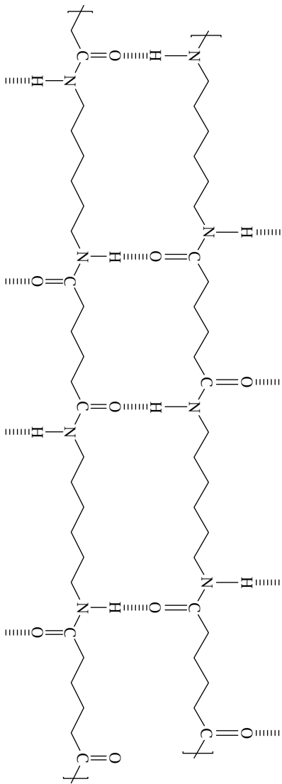
جزيئات بوليمرات نايون مرتبطة بروابط هيدروجين بعد إجراء عملية السحب على البارد
