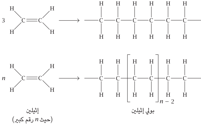
شكل ٢٦-١: ارتباط جزيئات الإيثيلين لتكوين بولي إيثيلين غير متفرّع.
