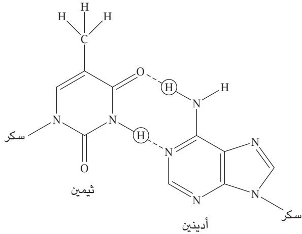
شكل ٣٤-٣: أزواج قواعد الأدينين والٲيمين والجوانين والسيٲوزين في صور التشكُّل الصحيحة.
