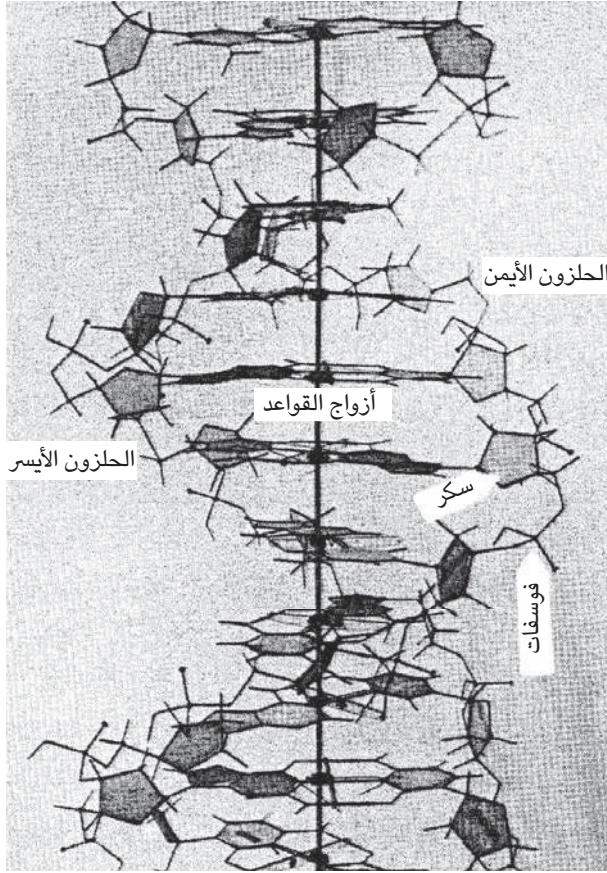
شكل ٣٤-٢: منظر جانبي لنموذج جزيء الحمض النووي.
