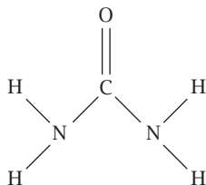
شكل ١٤-٤: الصيغة الجزيئية لليوريا.
