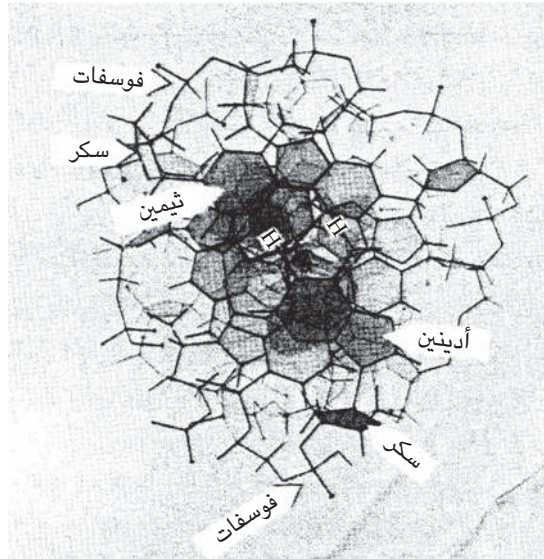
شكل ٢٤-١: منظر علوي لنموذج جزيء حمض نووي. قارنه بشكل ٣٤-٢.
