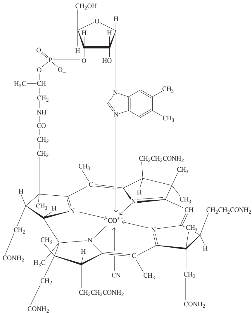
شكل ٩-١: الصيغة الجزيئية لفيتامين ب١٢.
