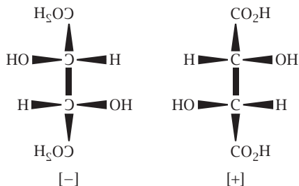
شكل ١٢-٤: شكلا حمض الطرطير في الجانبين الأيمن والأيسر (صورة مرآوية مطابقة).
