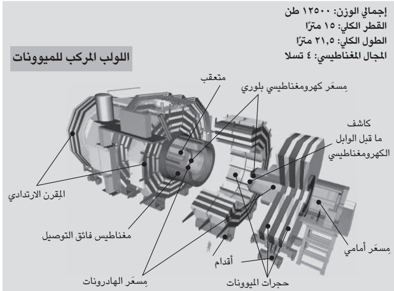
شكل ١٣-٥: صورة بالكمبيوتر للؤلؤ المركب للميونات مُفكَّكًا لعرض كلِّ مكوّن من مكونات الكاشف (الرسم مُقدّم من سيرن وتجربة اللؤلؤ المركب للميونات).
