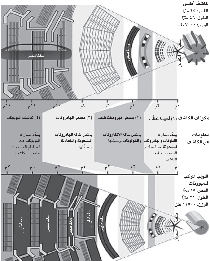
شكل ١٢-٤: مقاطع عرضيّة لكاشفَي أطلس واللولب المركب للميونات. يُرجى ملاحظة أن الأحجام الكلية بالرسم لا تعبّر عن الأحجام الحقيقية.
