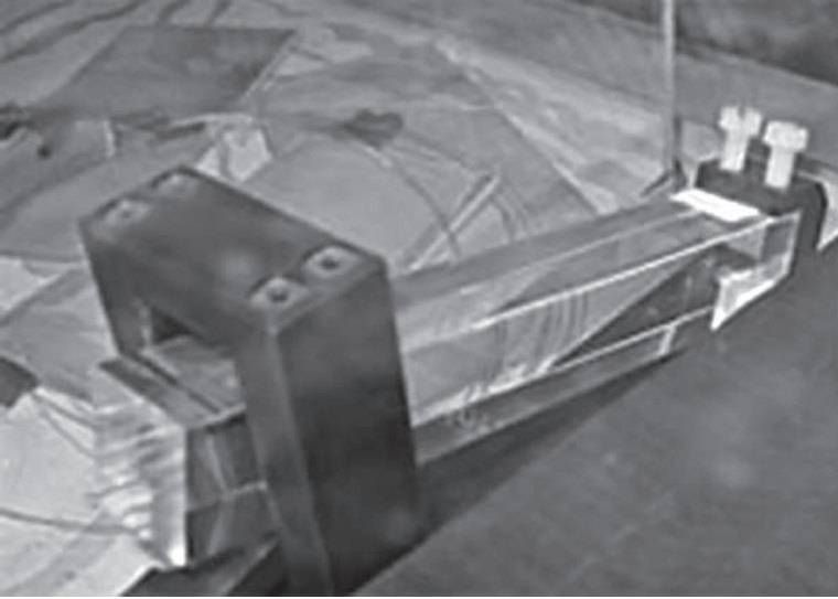
شكل ١٣-٨: صورة فوتوغرافية لبلورة تنجستات الرصاص المُستخدَمة في المُسرِّع الكهرومغناطيسي بالولب المركب للميونات.
