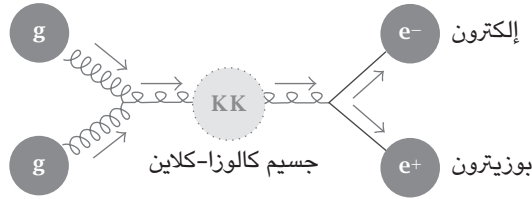
شكل ١٧-١٤: في نماذج راندل-ساندرم، يمكن أن ينتج جرافيتون كالوزا-كلاين ويتحلل داخل الكاشف إلى جسيمات مرئية، مثل الإلكترون والبوزيترون.
