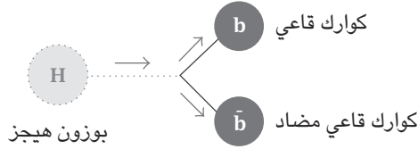
شكل ١٦-٣: سيتحلل بوزون هيجز الخفيف في الغالب إلى كواركات قاعية.
