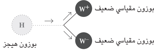
شكل ١٦-٢: يمكن لبوزون هيجز الثقيل أن يتحلل إلى بوزونات W القياسية.
