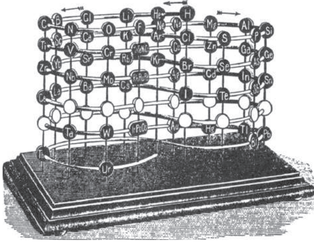
شكل ٤-٥: لولب وليام كروكس التلوري؛ وهو نموذج بديل بدائي من الجدول الدوري.
