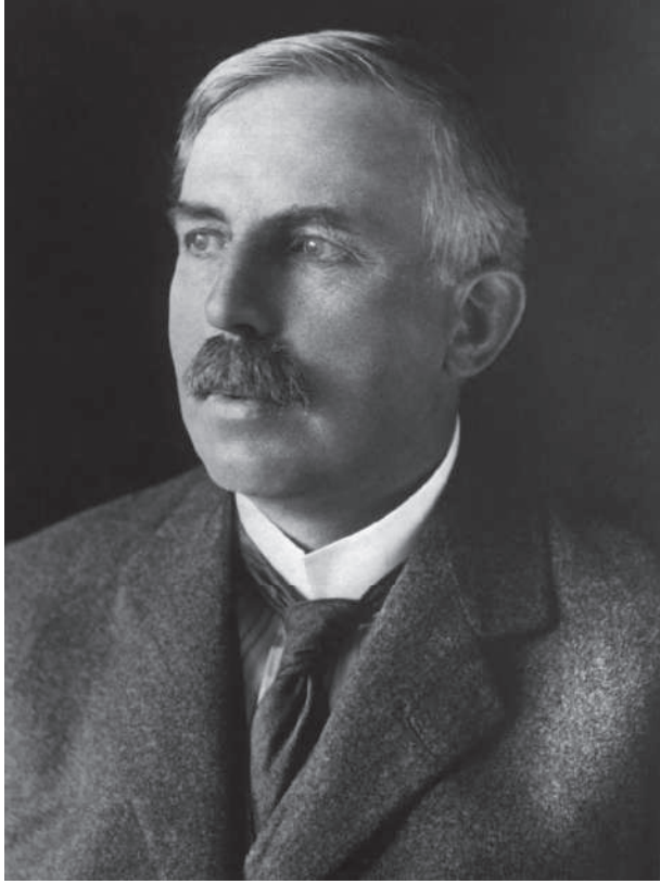
شكل ١-٥: استنتج إرنست رذرفورد (١٨٧١-١٩٣٧م) البنية الأساسية للذرات وأنشأ مجال الفيزياء النووية.
