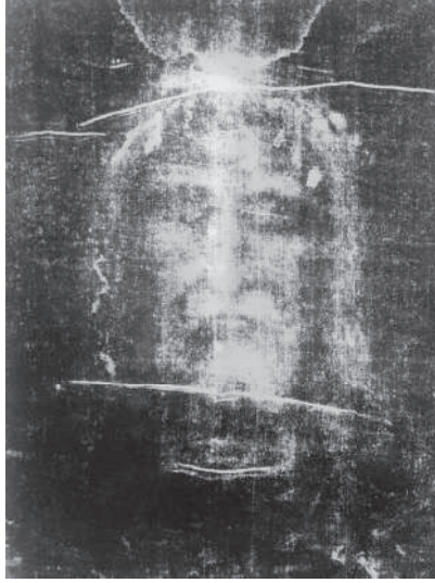
شكل ٦-١: التأريخ بالكربون المشع لكفن تورينو يشير إلى أنه صُنِعَ في القرن الثالث عشر أو الرابع عشر.
