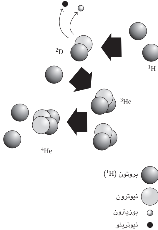
شكل ٥-٢: اندماج ذرّات الهيدروجين في الشمس يشكّل الهليوم ٤ ويطلق كمية هائلة من الطاقة.
