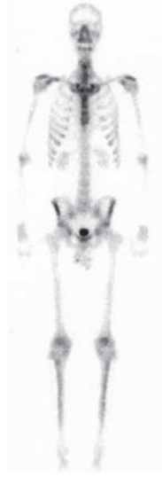
شكل ٦-٣: صورة لجسم إنسان مسجلة من التحلل الإشعاعي للتكنيشيوم ٩٩ شبه المستقر في مجرى الدم.
