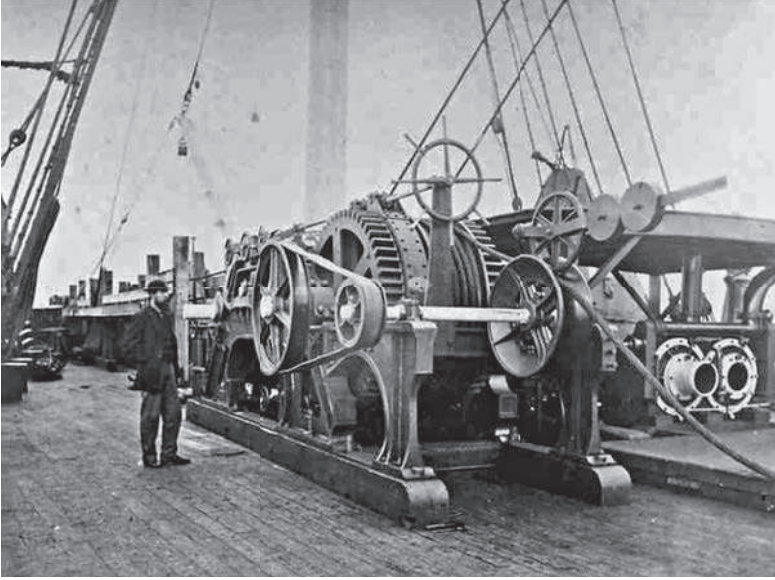
شكل ٧-٥: آلة مدّ الكابل التي كانت على متن السفينة جريت إيسترن في ١٨٦٦. قلّت آلية التلقيم المحسّنة من الضغط على الكابل أثناء مدّه إلى أعماق الأطلسي. المصدر: مكتبة الكونجرس الأمريكية.
