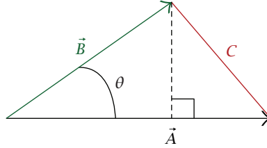
شكل ٨: قانون جيب التمام مطبق على الأطوال المتجهية.
