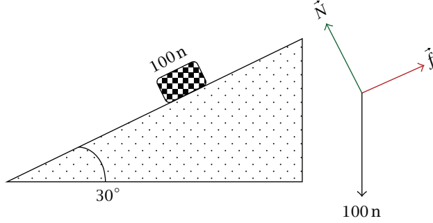
شكل ١٦-٢: الرسم التوضيحي ومخطط الجسم الحر لمثال ١٠-٢.
