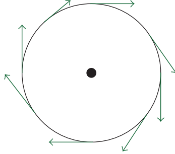
شكل ٨-٢٠: عجلة تدور حول محور خلال مركزها، أو عجلة تتدحرج بطول سطح مسطح كما يُرى من إطار إسناد متحرك مع مركز العجلة، ولها سرعات جزيء كما هو مبين.
