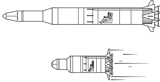
شكل ١-٥: من منظور مسئول المراقبة، لن يتقلص طول المركبة الفضائية وحده، بل ستتقلص كل محتوياتها أيضاً.
