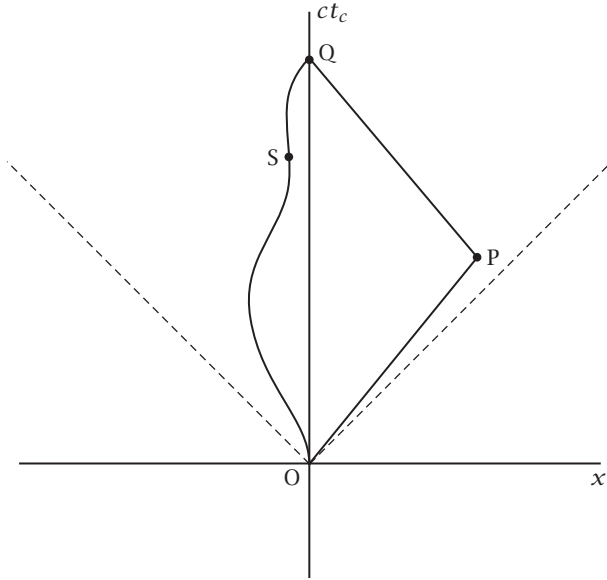
شكل ١١-٢: الخطوط العالمية الخاصة للتوأمين المشارك فيما يطلق عليه «معضلة التوأمين».
