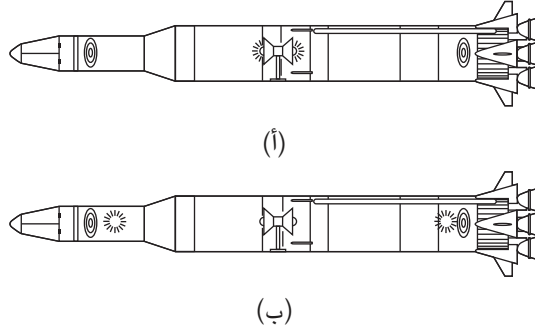
شكل ١-٦: من منظور رائد الفضاء، النبضتان المنطقتان في الآن عينه من منتصف المركبة تصلان إلى طرفي المركبة على نحو متزامن.
