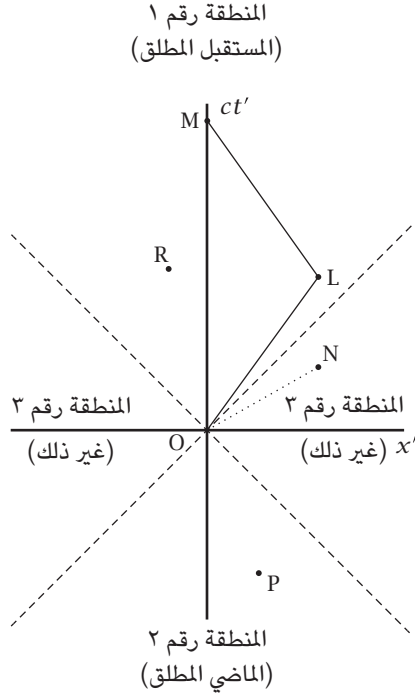
شكل ١-١٠: مخطط زمكاني يوضح المناطق الثلاث التي يمكن أن توجد بها الأحداث — المستقبل المطلق، والماضي المطلق، وغير ذلك — نسبة إلى الحدث O.
