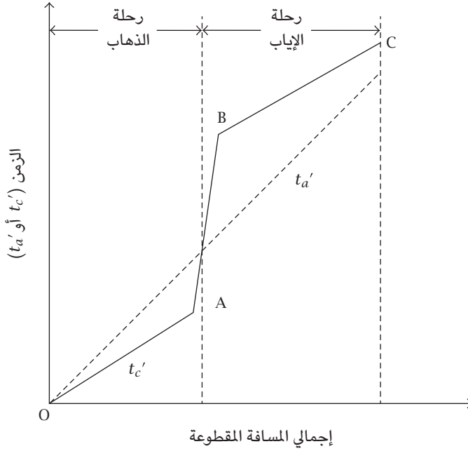
شكل ٢-٤: القراءة المسجلة على ساعة رائد الفضاء t_a' مقارنة بالقراءة المسجلة على ساعة مسئول المراقبة t_c' ، وذلك من منظور رائد الفضاء.
