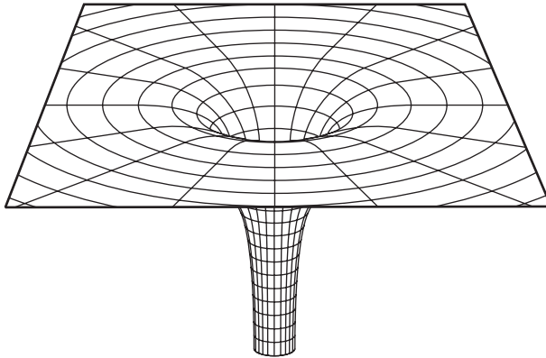
شكل ١٦-٢: منظر جانبي لانحناء الفضاء الذي يسببه ثقب أسود.
