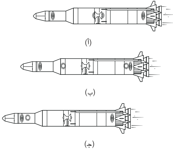
شكل ٧-١: من منظور مسئول المراقبة، النبضتان المنطقتان في الوقت عينه من منتصف المركبة لا تصلان إلى طرفي المركبة على نحو متزامن.
