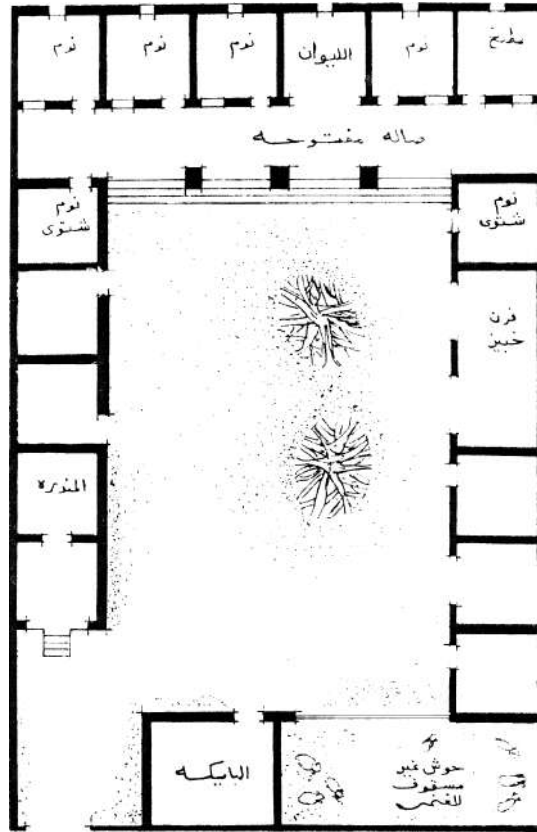
شكل ٨-١: مخطط المنزل العرايشي.
