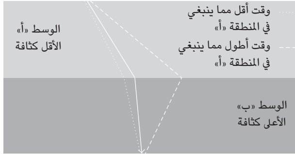
قانون سنيل
