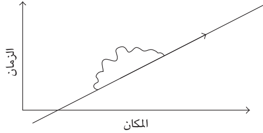
الطاقة الذاتية (إلكترون يتفاعل مع مجاله الكهرومغناطيسي)
