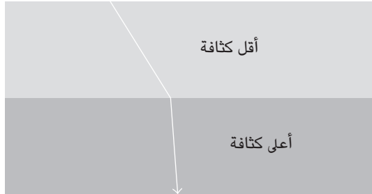
قانون سنيل
