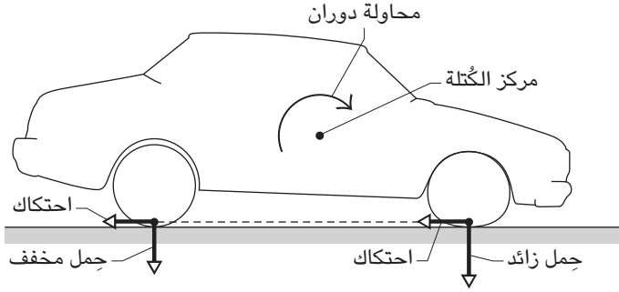
شكل ٣-١: بند ٧-١: سيارة تندفع إلى الأمام في أثناء الضغط على المكابح.
