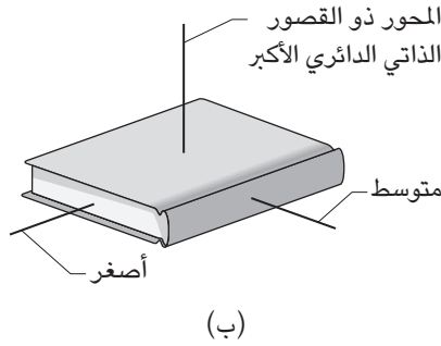
شكل ١-٣٥: بند ١-٩٦: (أ) ثلاثة محاور تمرُّ عبرَ الكتاب. (ب) القصور الذاتي الدائري المرتبط بالمحاور.
