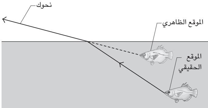
شكل ٦-٣٠: بند ٦-٨٤: موقع السمكة الظاهري والحقيقي.
