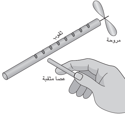
شكل ١-٥٤: بند ١-١٦١: تدور المروحة على طرف الدبوس بعد أن تهتز العصا.
