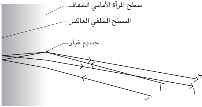
شكل ٤٢-٦: بند ١١٠-٦: طريقان لتشتت الضوء إلى المشاهد من جسيم غبار أمام مرآة.
