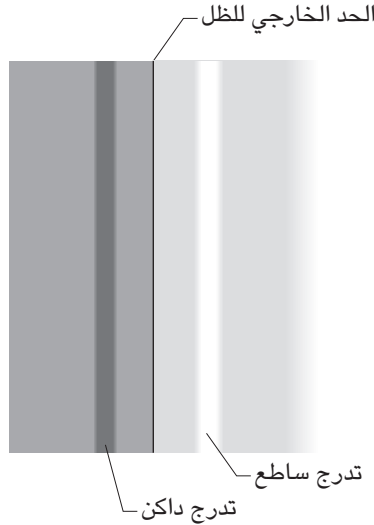
شكل ٥-٧: بند ٧-٢٥: تدرجات ماخ اللونية عبر الحد الخارجي للظل.
