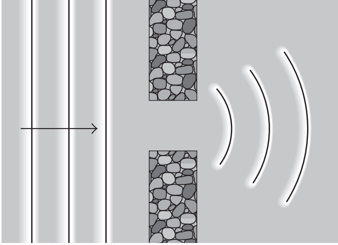
شكل ٢-٢١: بند ٢-٦٦: منظر علوي لأمواج محيط تتعرّض للحيود من خلال فتحة في جدارٍ صخري.
