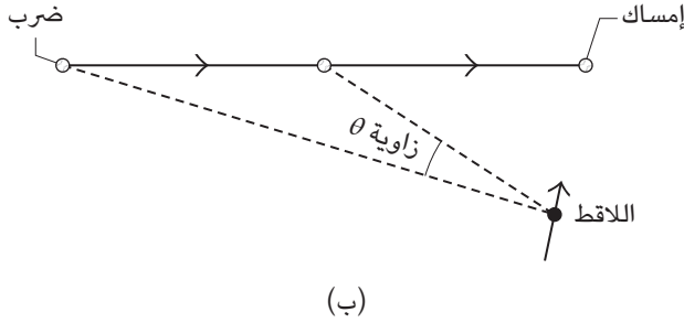
شكل ١-٦: بند ١-٢١: (أ) منظر جانبي لمسار الكرة الطائرة. (ب) منظر عمودي للمسار.
