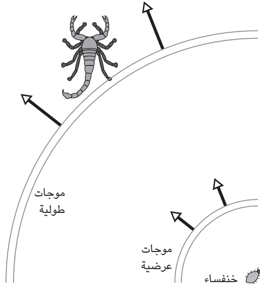
شكل ١-٤٥: بند ١-١٢٧: موجات تُنبّه العقرب بحركة الخنفساء.
