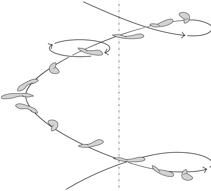
شكل ٣-٢: بند ١١-٢: مسار مُحتمَل لبذرة مُجنَّحة تدور عكس اتجاه الدوران في مسار لولبي.
