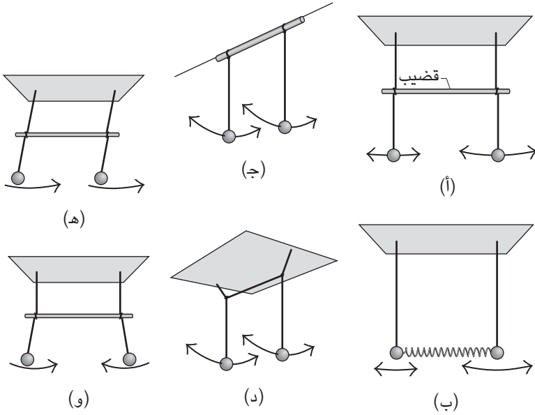
شكل ١-٤٢: بند ١-١١٩: (أ)-(د) بندولان مُقترنان. (ه)-(و) نمطان عاديان للحركة.
