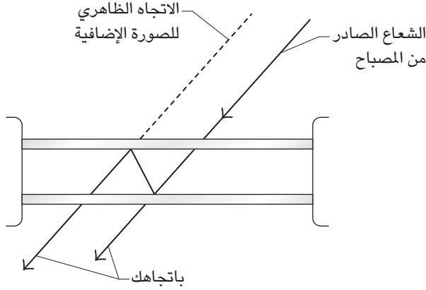
شكل ٦-٢٩: بند ٦-٧٩: مسار الضوء عبر نافذة مزدوجة.
