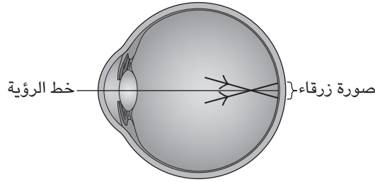
شكل ٧-٨: بند ٧-٤٣: عندما تركز العين على النقطة الحمراء بشدة، فإنها تركز النقطة الزرقاء أمام الشبكية.
