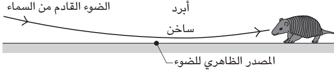
شكل ٩-٦: بند ٦-٢٨: مسار الضوء من السماء المُنخفضة وانكساره بفعل التغير في درجة حرارة الهواء. يرى المراقب أن مصدر الضوء يأتي من الأرض.
