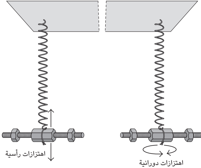
شكل ١-٥٠: بند ١-١٥٠: بندول ويلبرفورس يُبادل بين الاهتزازات الرأسية والاهتزازات الدورانية.
