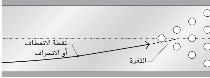
شكل ١-٢٧: بند ١-٧٣: مسار كرة البولينج.
