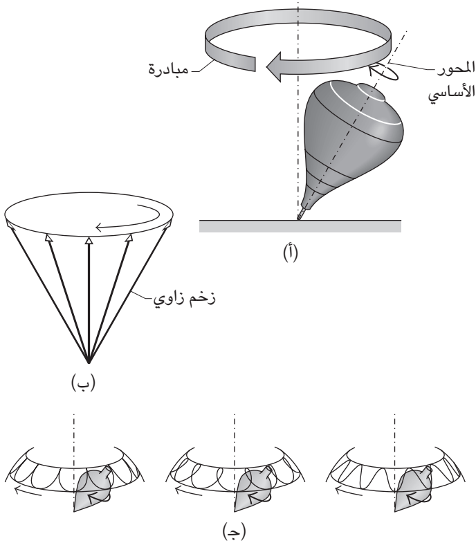
شكل ١-٣٧: بند ١-١٠٤: (أ) حركة مبادرة لعبة النحلة حول محور رأسي عبر نقطة التماس (ب) يتحرك مُتَجِّه الزخم الزاوي للعبة النحلة حول المحور الرأسي (ج) التمايل أثناء حركة المبادرة.
