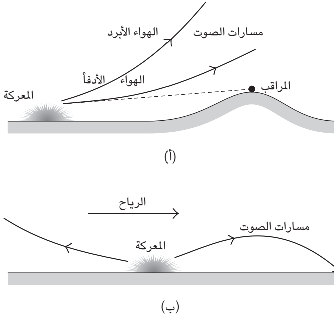
شكل ٣-٣: بند ٣-١٩: (أ) يحدث انحناء للصوت القادم من المعركة بعيداً عن المراقب في حالة انخفاض درجة حرارة الهواء مع الارتفاع. (ب) تعمل الرياح على انحناء مسارات الصوت.
