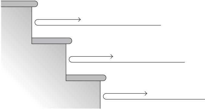
شكل ٦-٣: بند ٣-٦٥: انعكاسات الصوت من درجات السلم.
