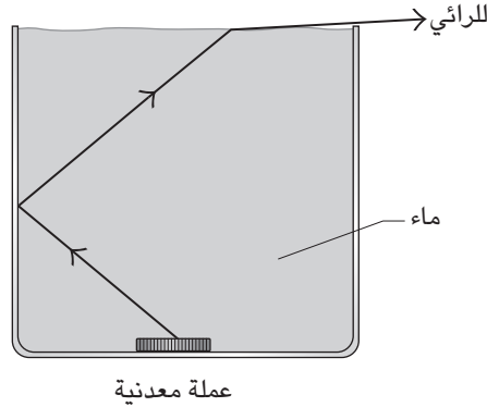
شكل ٦-٤٩: بند ٦-١٣٨: عملة معدنية تُرى عبْر سطح الماء داخل البرطمان.
