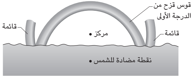
شكل ٦-٢: بند ٦-٢: يستطيع الضوء الذي يعكسه الماء أن يُشكّل قوس قزح، مركزه نقطة أعلى من قوس قزح الدرجة الأولى. هنا، تظهر قائمتا قوس قزح الإضافي فقط.
