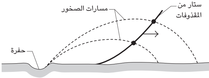
شكل ١-١٢: بند ٣٧-١: صخور مُتناثرة من جراء اصطدام نيزك بالأرض.
