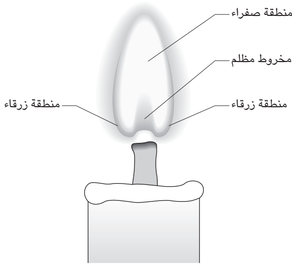
شكل ٤-١٢: بند ٤-٧٨: تركيب لهب الشمعة.
