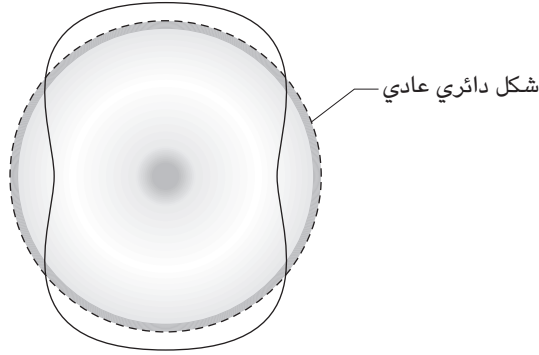
شكل ٤-٣: بند ٤٣-٣ و ٤٤-٣: صورة فوقية مكبرة لحافة كأس خمر مُهتزة.
