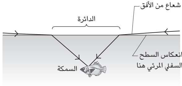
شكل ٦-٣١: بند ٦-٨٥: الضوء الخارجي يصل إلى السمكة عبر دائرة فوقها.
