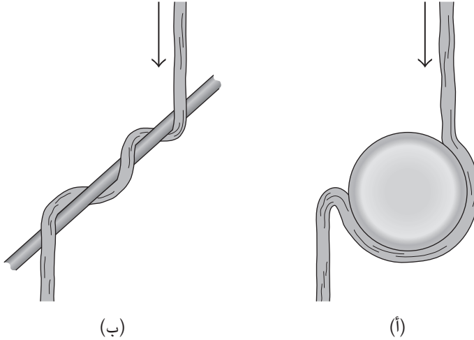
شكل ١٦-٢: بند ٢-٥٠: تيار ماء ساقط يلتف حول (أ) برطمان، و(ب) قضيب مائل.
