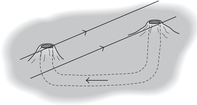
شكل ٨-٢: بند ٢-٢٢: رياح تمر عبر تَلَّتَيَّ أحد جحور كلب البراري.
