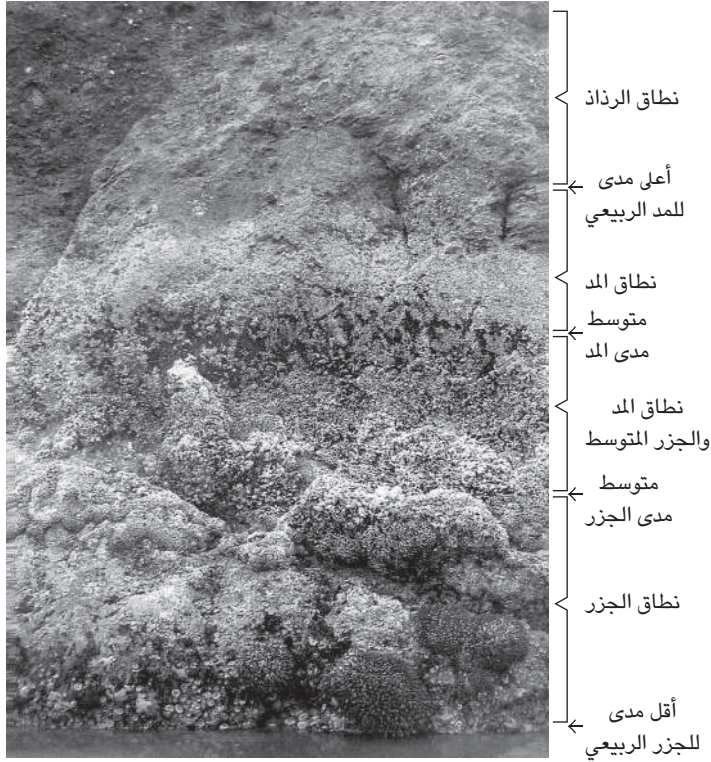
شكل ٧-١: نمط نموذجي لتقسيم مناطق المد والجزر في حالة الجزر على شاطئ صخري في ولاية واشنطن بالولايات المتحدة الأمريكية.
