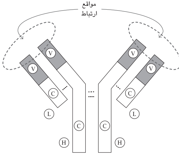
شكل ٣-٤: يتكوّن جزيء الجلوبيولين المناعي من سلسلتين ثقيلتين (H) واثنيتين خفيفتين (L) من عديدات الببتيد تُشكل هيكلًا على شكل حرف Y بطرف ثابت (C) وموقعين مُتغيّرين لارتباط الأنتيجين (V).
