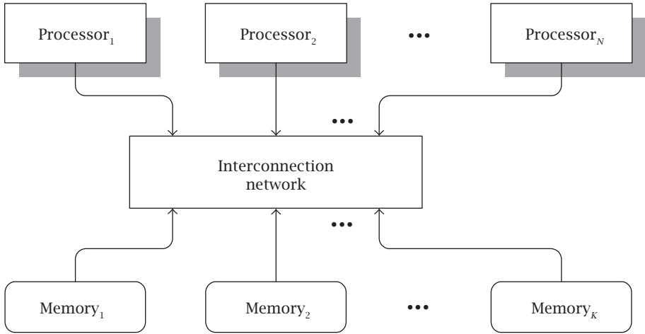
شكل ٥-٤: مخطط معالج متعدد.
