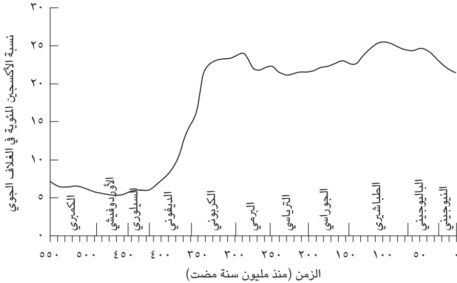
شكل ٣-٣: تنظيم نسبة الأكسجين في الغلاف الجوي على مدار حقبة الفانيروزوي. نتائج مأخوذة من نموذج «كوبس».
