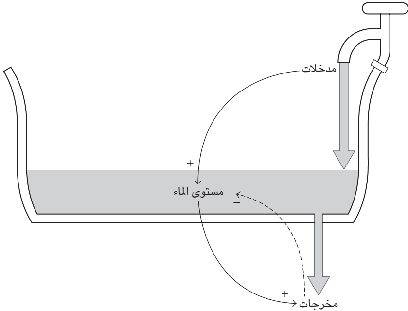
شكل ٣-١: شكلٌ يوضح تشبيه عملية التنظيم والتحكم بحوض استحمام. تتحكم التغذية المرتدة السالبة في كمية المواد التي تخرج من المخزن.
