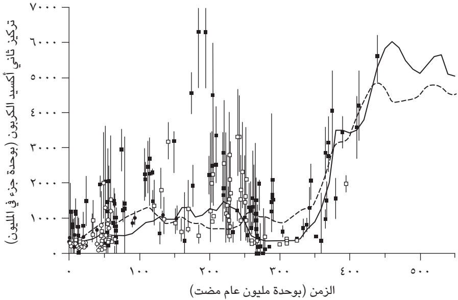
شكل ٣-٤: تباين تركيز ثاني أكسيد الكربون في الغلاف الجوي على مدار حقبة الفانيروزوي. مجموعة مُجمّعة من بياناتٍ بديلة (نقاط ذات نطاقات خطأ) وتنبؤات نموذجية (تنبؤات نموذج «جيوكارب ٢» مُمثلة بالخط المتصل، وتنبؤات نموذج «كوبس» مُمثلة بالخط المتقطع).
