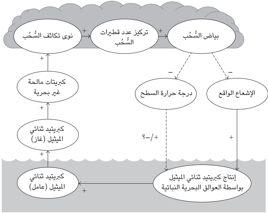
شكل ٥-٣: فرضية «سي إل إيه دبليو» لآليات التغذية المرتدة بين إنتاج كبريتيد ثنائي الميثيل ولبياض السحب والمناخ.
