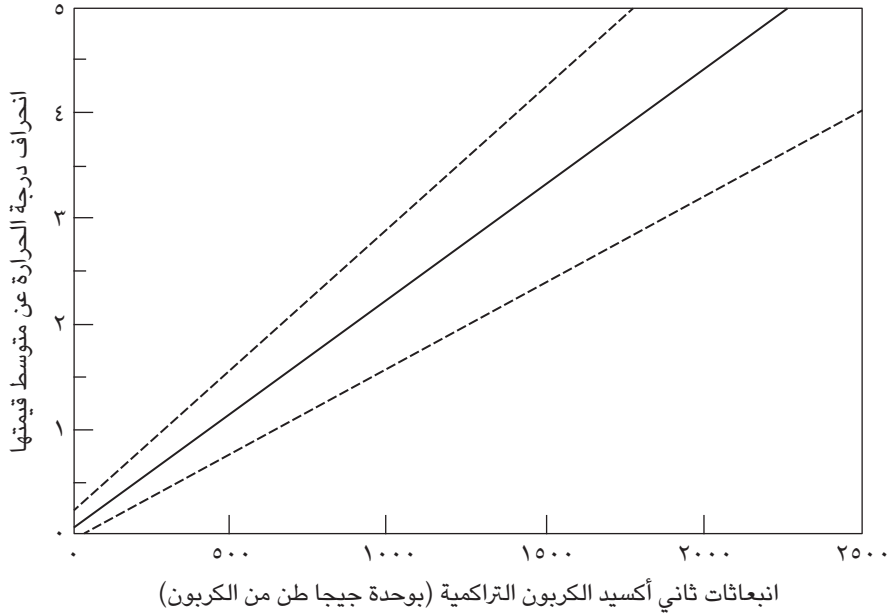
شكل ٦-١: العلاقة بين انبعاثات الكربون التراكمية والتغير العالمي في درجة الحرارة من مجموعة من نماذج نظام الأرض الحديثة.
