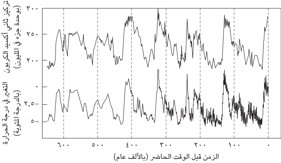
شكل ٦-٣: سجل العينة الأسطوانية الجوفية المأخوذة من القارة القطبية الجنوبية المُعبّر عن تغيّر تركيز ثاني أكسيد الكربون في الغلاف الجوي ودرجة الحرارة (رُسم هنا بمقياس مُعدّل ليعبّر عن تغيّر درجة الحرارة على مستوى شبه عالمي).
