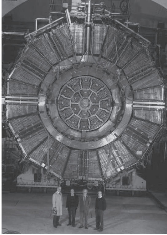
شكل ٦-٥: أحد الكواشف في مصادم الإلكترونات-البوزيترونات الكبير وإلى جواره أربعة من العلماء، ويتضح من الصورة حجم الكاشف. 4
