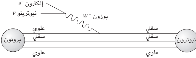
شكل ٧-٢: تحلل بيتا عن طريق البوزون W^- : يتحول النيوترون إلى بروتون عن طريق إطلاق بوزون W^- ، الذي يتحول بعد ذلك إلى إلكترون ونيوترينو.
