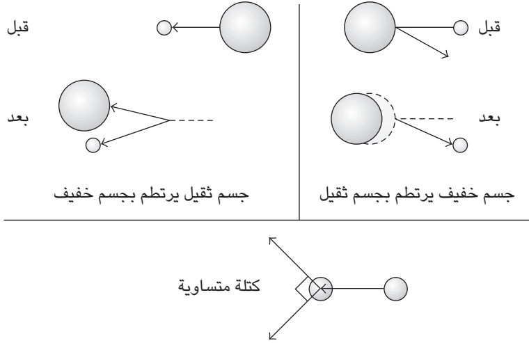
شكل ٣-١: نتائج ارتطام الأجسام الثقيلة والخفيفة بالأجسام الخفيفة والثقيلة، على الترتيب.
