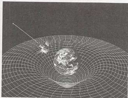
شكل ثنائي الأبعاد يصور تحذب الفضاء نتيجة لتشويش وجاذبية الأجسام للفرغ
