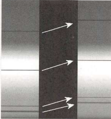
الانزياح الأحمر للضوء بفعل سرعة المصدر في الابتعاد عنا. الانزياح نحو الأحمر معناه زيادة طول موجة الضوء القادم إلينا، طبقاً لظاهرة دوبلر
