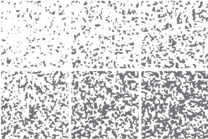
محاكاة لتطور البرك الذائبة بناءً على نموذج إيزينج.
