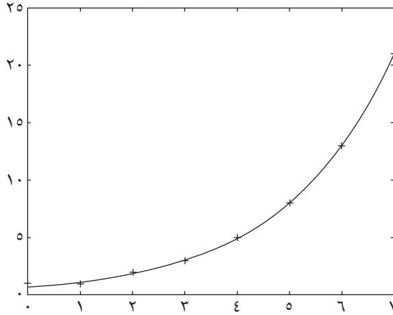
شكل ٢-١: سلسلة صلبان تُظهر عدد أزواج الأرانب شهرياً (أرقام فيبوناتشي)؛ ويمثل المنحنى البسيط الذي تقع الصلبان قرب نموها الأسّي.
