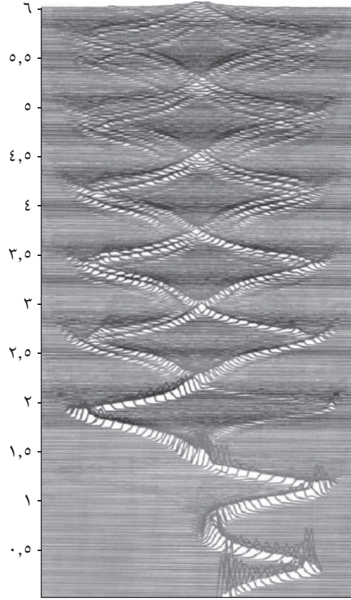
شكل ٤-٥: التوقع الاحتمالي الذي قد يضعه شيطان القرن الحادي والعشرين في نظام لورنز الذي وضعه في عام ١٩٦٣. قارن بين الطريقة التي يتطور بها عدم اليقين في هذا النظام الفوضوي مع الزيادة البسيطة نسبياً في عدم اليقين في خريطة يول الموضحة في الشكل رقم ٣-٤.
