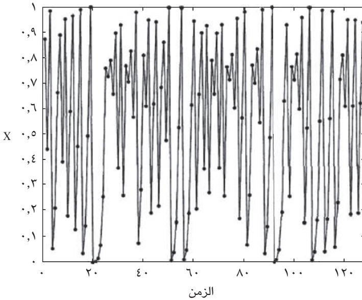
شكل ٣-١: سلسلة زمنية فوضوية مستقاة من الخريطة اللوجستية الكاملة التي تبدأ قرب قيمة X_0 تساوي ٠,٨٧٦. لاحظ أن السلسلة قابلة للتوقع بصورة واضحة متى كانت قيمة X تقترب من الصفر و 3/4 .
