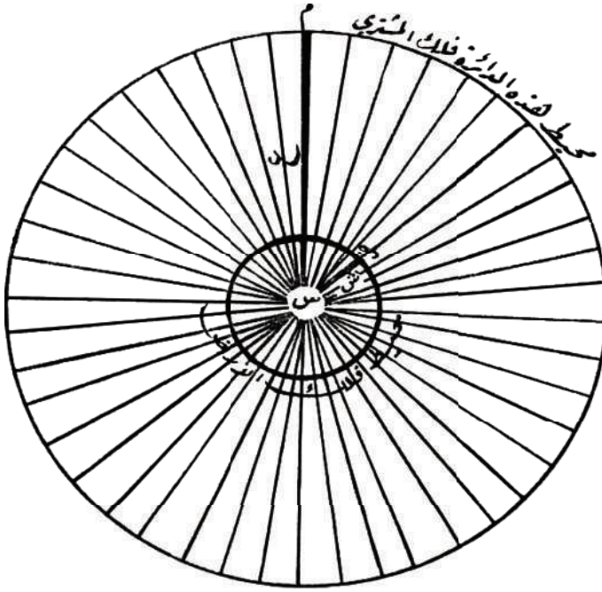
شكل ٢: الخطوط الصادرة من مركز الدائرة (الشمس) هي خطوط القوة (الجاذبية).
