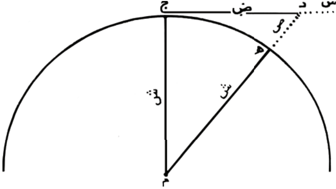
شكل ١: الشعاعان ش ش منفرجان أكثر من اللازم للتمكن من رسم الأحرف الرمزية.
