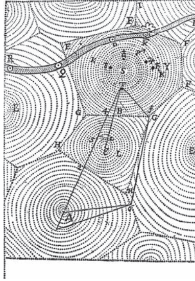
شكل ٣-١: نظرية الدوامات الديكارتية: النظام الشمسي، المحيط بالشمس (S)، ويحده النقاط FFFFGG. أما النظام الأخرى فتحتوي نجومًا في مركزها.
